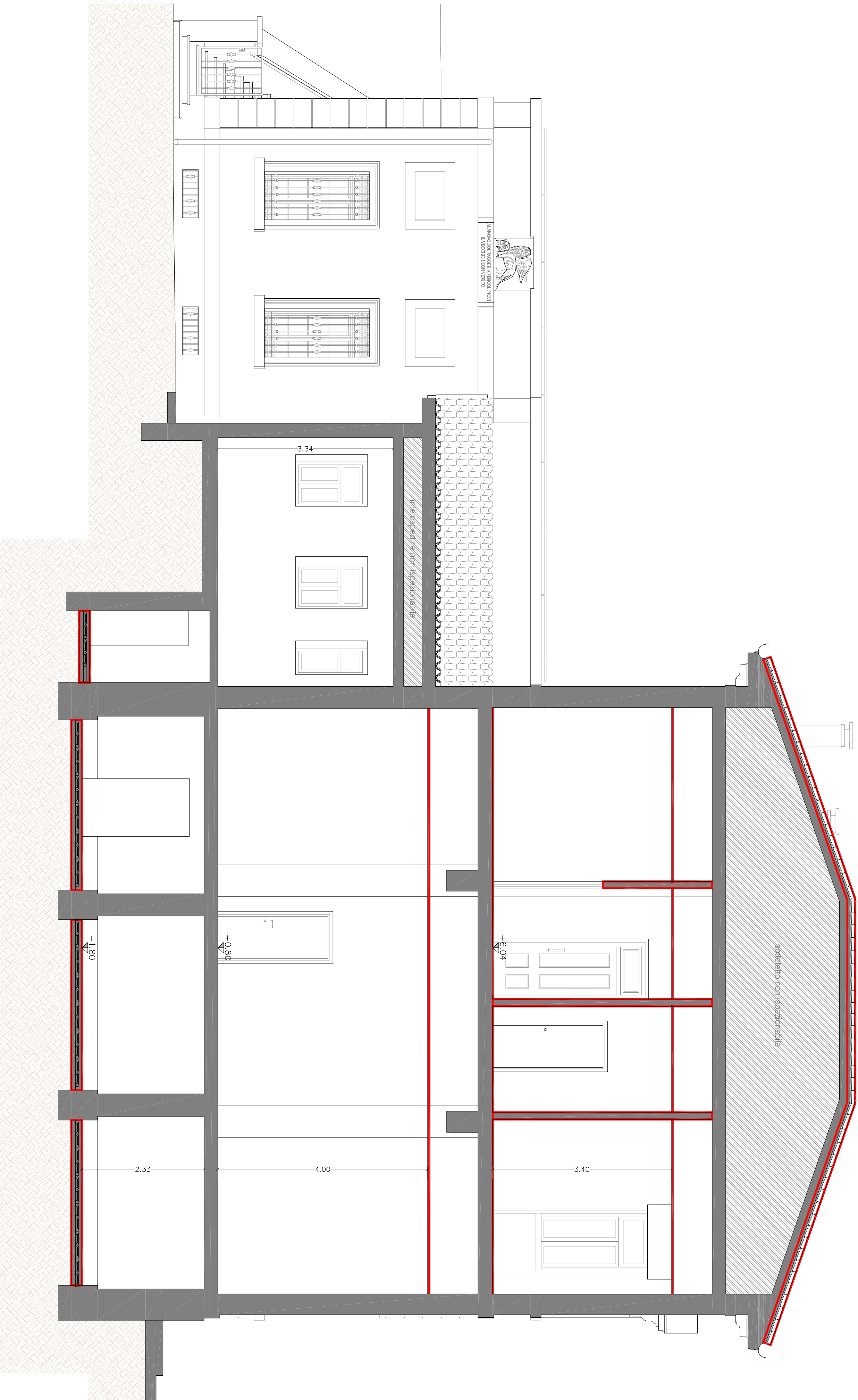
SEZIONE AA - STATO DI PROGETTO
