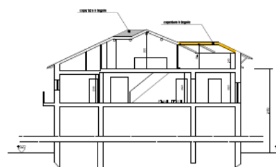
Sezione A-A
