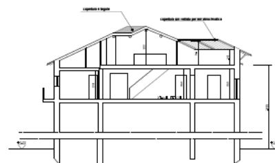
Sezione A-A
