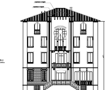
Prospetto sul giardino prospiciente Via Caprera
