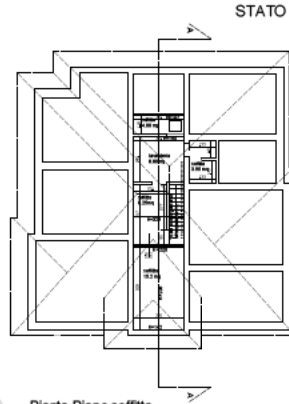
Pianta Piano soffitta
