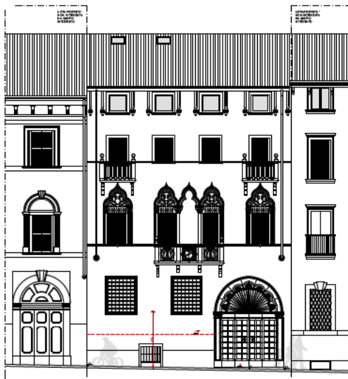
PROSPETTO SU VIA RANGINI - SCALA 1:50
