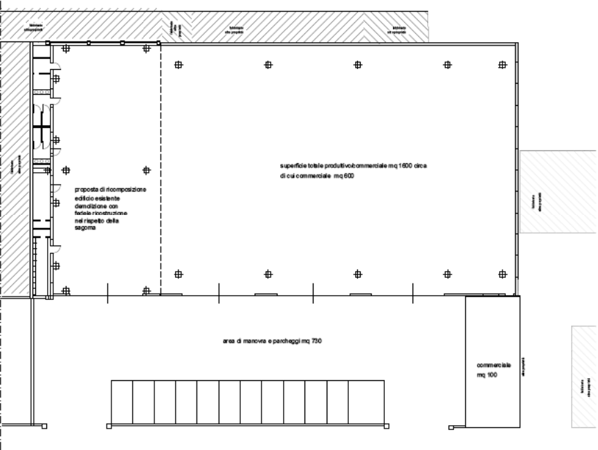
Pianta Piano terra proposta indicativa di progetto 1:100
